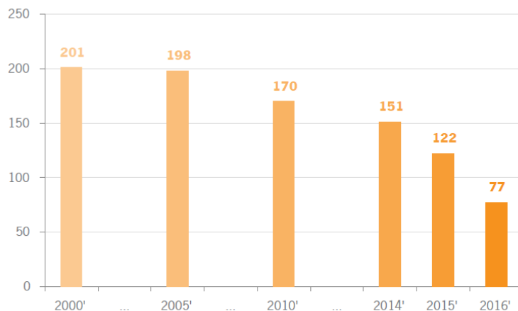
Wykres 2. Średni okres prac nad ustawą (od wpłynięcia do Sejmu do podpisu Prezydenta; w dniach)
