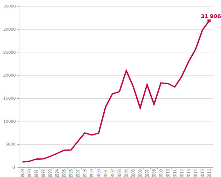
Wykres 1. Liczba stron aktów prawnych przyjmowanych w poszczególnych latach – od 1989 r.
